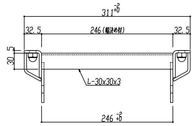
巾決め取付要領図
